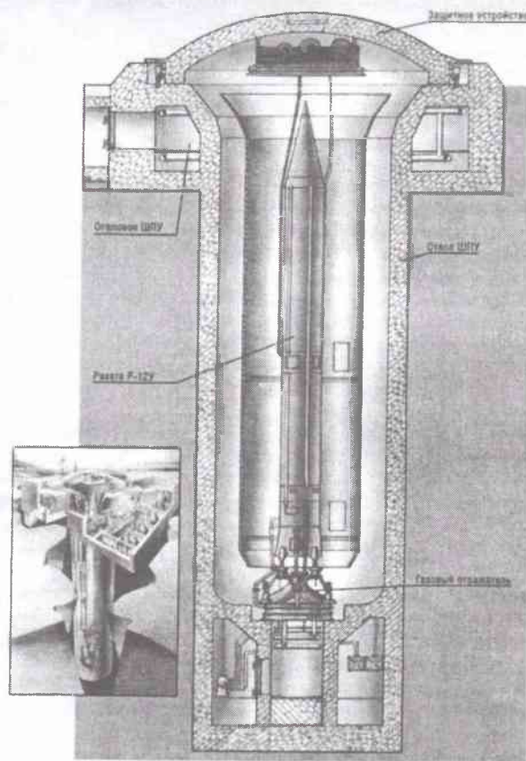
Шахтная пусковая установка Р12У
