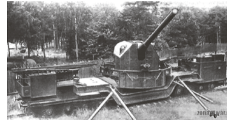
ТМ-1-180 – железнодорожная артиллерийская система
