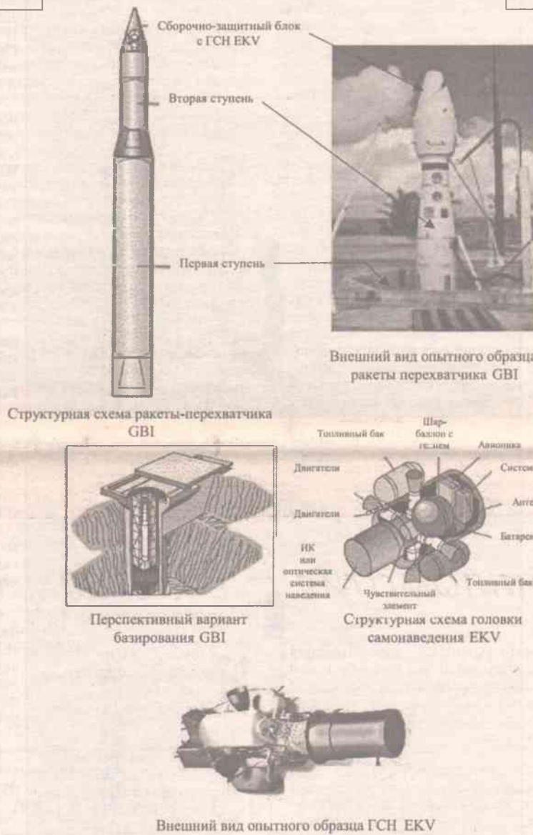
Рис.3. Ракета-перехватчик GBI и головки самонаведения EKV – структурные схемы и опытные образцы
