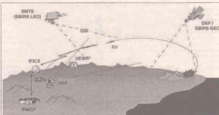
Рис.4. Схема функционирования перспективной НПРО США и взаимодействие ее составных элементов
