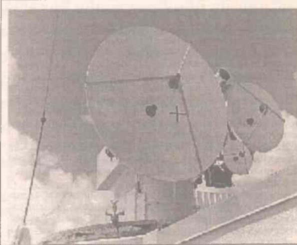
Рис.2 Внешний вид опытного образца станции поддержания связи с перехватчиком в полете (IFICS)
